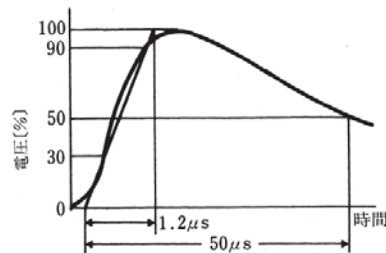
電圧出力端子開放における電圧サージであつて、ピーク値は1kV
